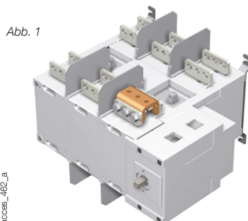
Oben oder unten Flachanschluss
