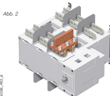
Oben oder unten Hochkantanschluss
