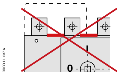
SIRCO PV 037 A Das Design anderer Hersteller mit einer kürzeren Luftstrecke. Die Klemmenabdeckungen verlängern diese Strecke nicht.
