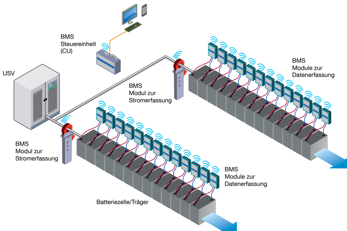
Drahtloses Funk-Batterieüberwachungssystem.
