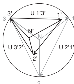
Unsymmetrisches Netz
