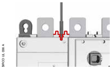
SIRCO UL 036 A SOCOMEC-Ausführung: Luftstrecke 53 mm (außen und innen)
