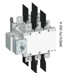
SIRCO PV 800 A 1500 VDC mit zwei Lasttrennschaltern 400 A in Back-to-Back Version.
