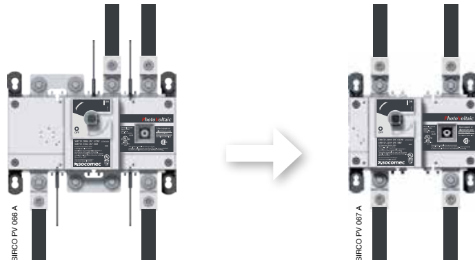
Klassische Lösung Beispiel des Anschlusses eines Schalters für 1000 VDC.
