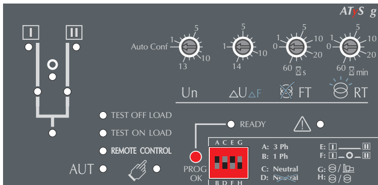
Vorderseite des Steuerrelais
