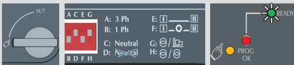
MÖGLICHE DIP-SCHALTEREINSTELLUNGEN
